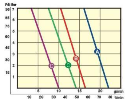
HD-A16: A-7bar B-4bar HD-A6: C-7bar D-4bar
